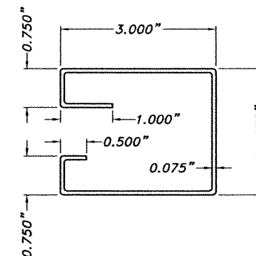
4 ROLLFORMED GUIDE SCALE : N.T.S
