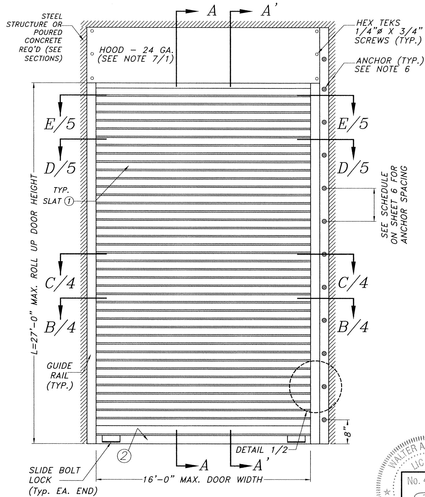
TYPICAL DOOR ELEVATION N. T. S.
